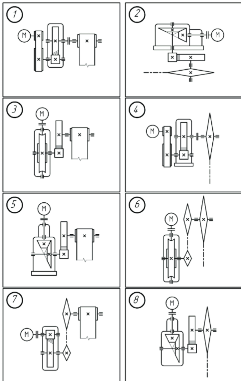
Рис. 1.1. Варианты кинематических схем, лист 1
