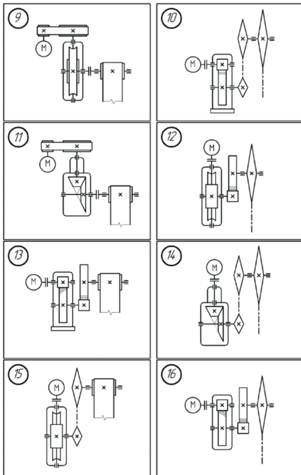
Рис. 1.1. Варианты кинематических схем, лист 2
