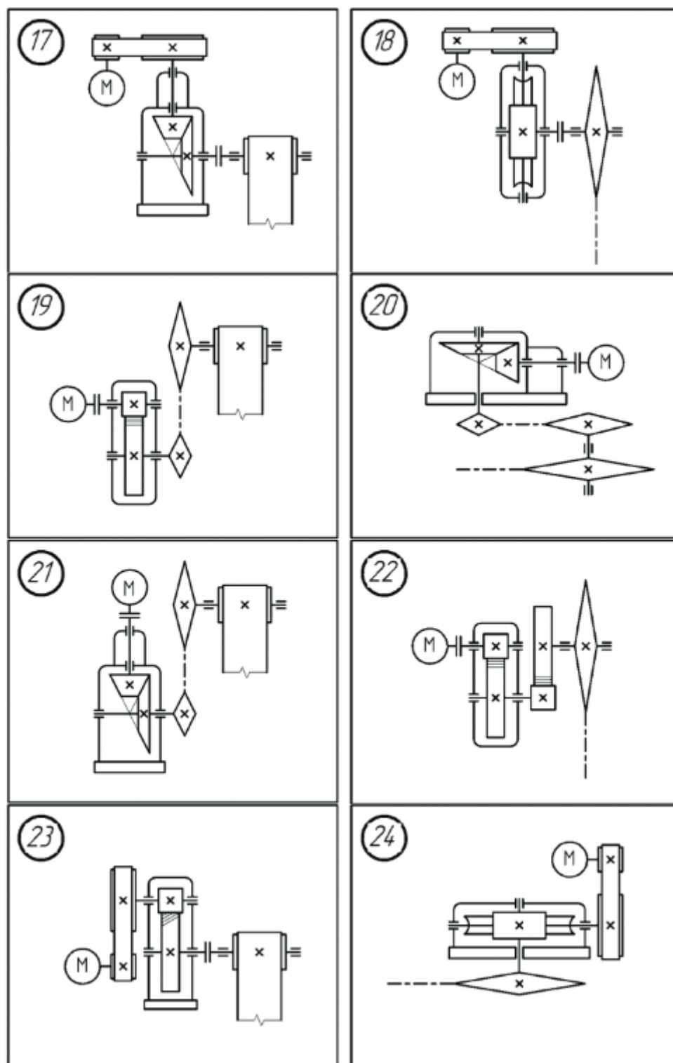
Рис. 1.1. Варианты кинематических схем, лист 3
