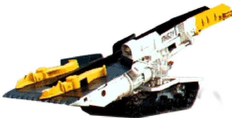
Рис. 4.10 Погрузочная машина 1 ПНБ-2У на гусеничном ходу, может использоваться при проходке горизонтальных и наклонных (до 18°) выработок
