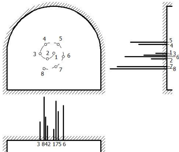
Рис.3.3. Спиралевидный вруб
