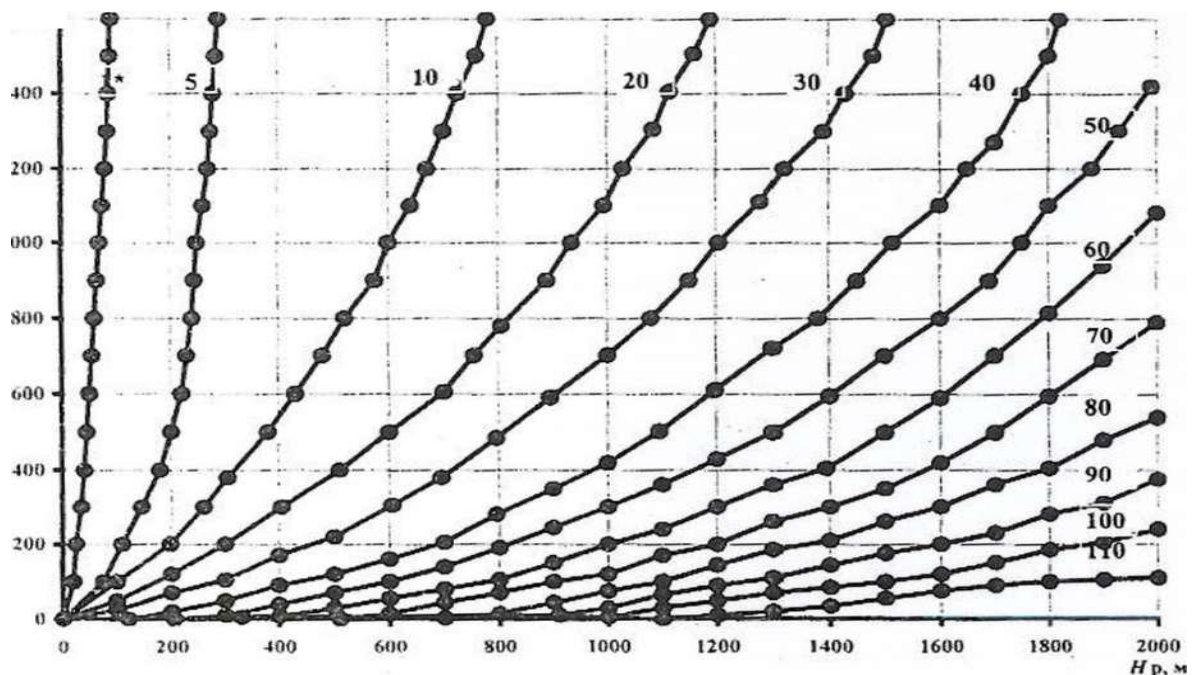
Рис.1.1. Графики для определения типового смещения пород u_t
