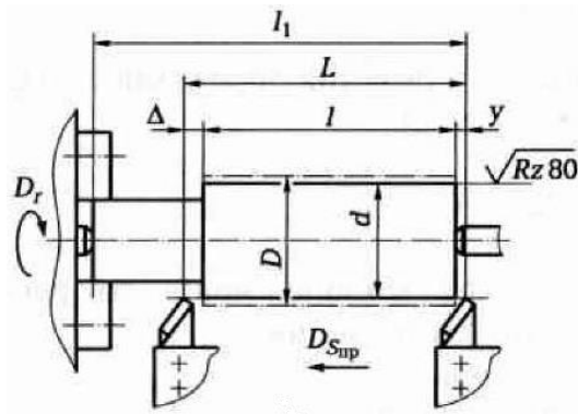
Рис. 1. Эскиз обработки
