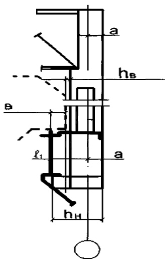
Рис. 4.8. Узел опирания подкрановой балки
