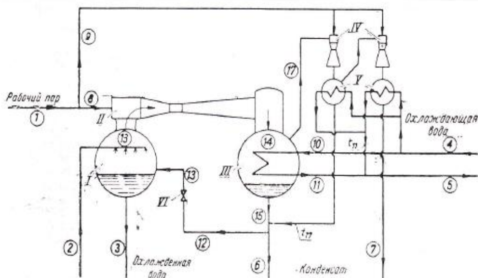
Схема парозжекторной холодильной установки. I — испаритель; II — основной эжектор; III — основной конденсатор; IV — вспомогательные эжекторы; V — вспомогательные конденсаторы; VI — дроссельный вентиль.
