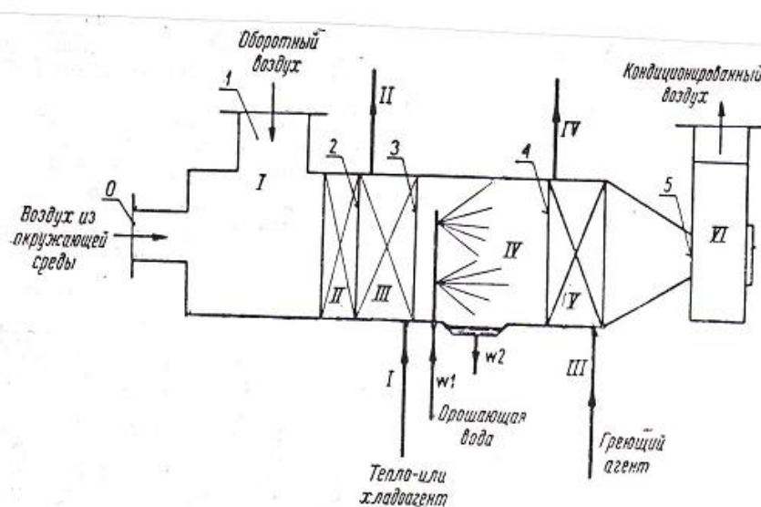
Схема кондиционирующего оборудования. I — смешивательная камера; II — фильтр; III — предварительный теплообменник; IV — камера орошения; V — конечный теплообменник; VI — вентилятор.
