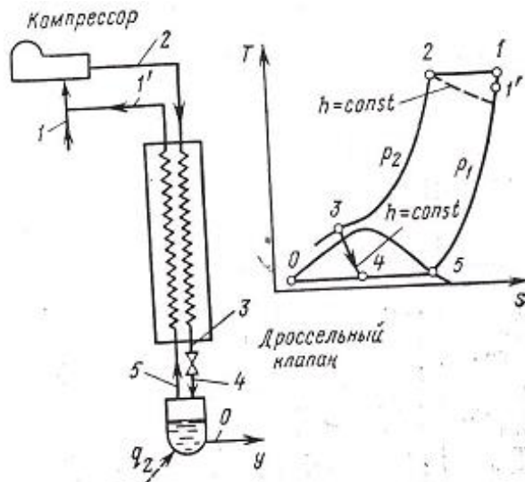
Рис. 8.4 Схема цикла с однократным дросселированием
