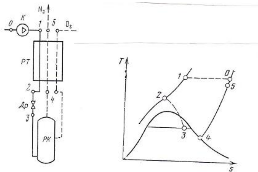
Схема простейшей ВРУ и ее цикл на диаграмме Т- s : 0...5 – точки процесса; К – компрессор; РТ – рекуперативный теплообменник; РК – разделительная колонна; Др – дроссель.
