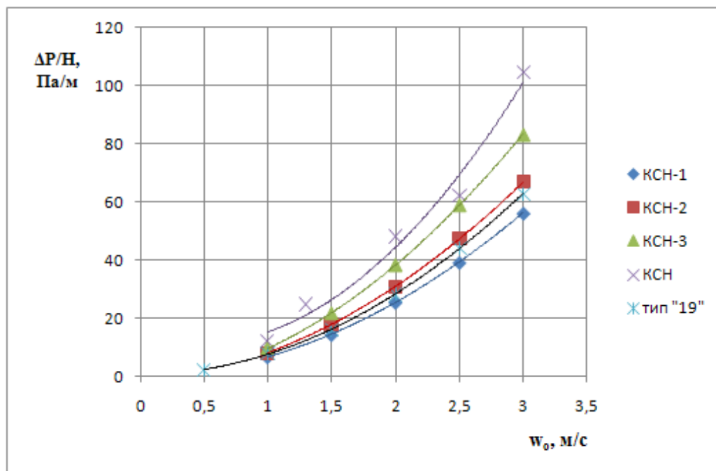
Рис. 3.4.3.1. Зависимость гидравлического сопротивления сухих (при q = 0 \text{ м}^3/(\text{м}^2 \cdot \text{ч}) ) насадок KCH-1, KCH-2, KCH-3, KCH и насадки типа «19» высотой блока H = 0,91 \text{ м} от скорости воздушного потока
