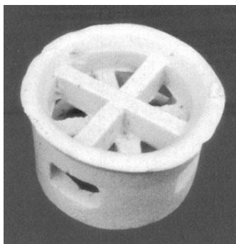
Рис. 4.4.7. Мини-кольцевая насадка
