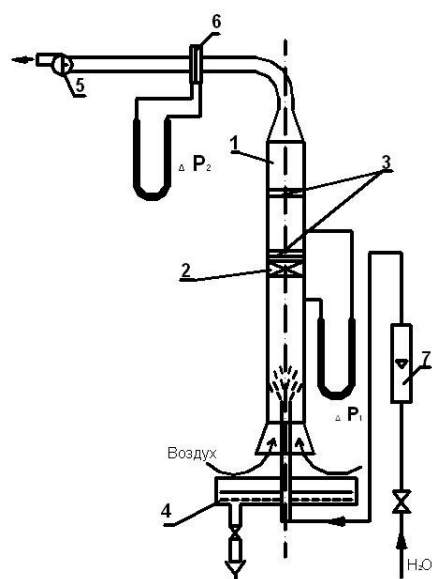
б) схема стенда
