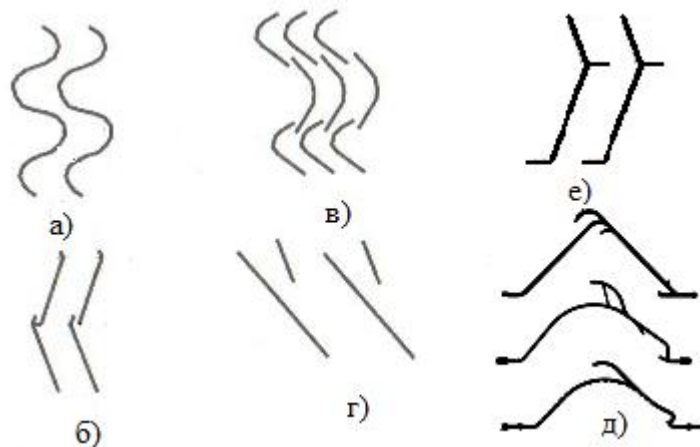
Рис. 4.3.3. Профили жалюзийных каплеуловителей:
