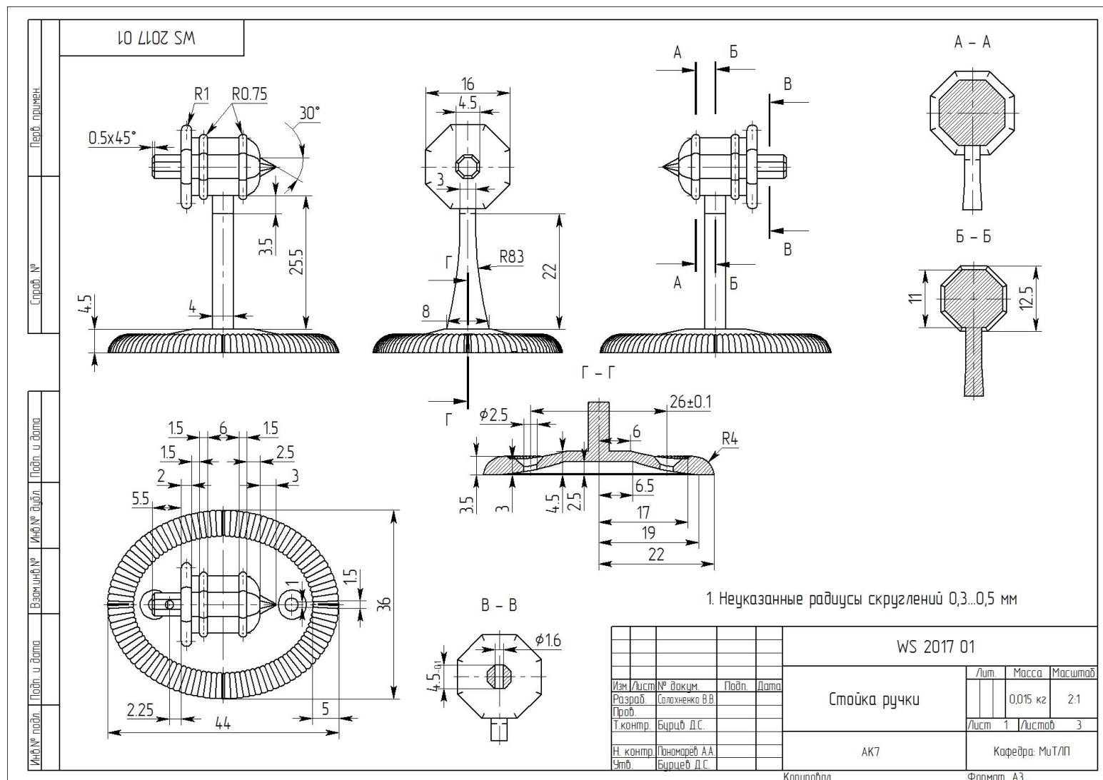
Рисунок 5. Чертеж стойки ручки (М1).
