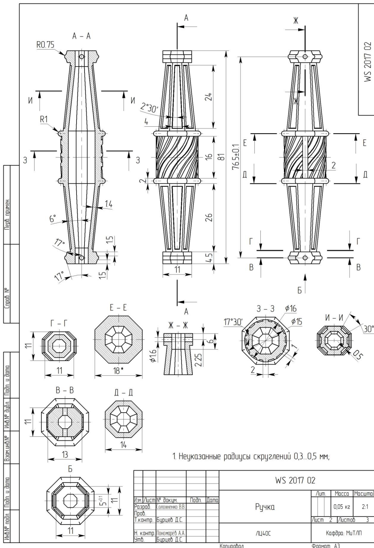
Рисунок 6. Чертеж ручки (М2).
