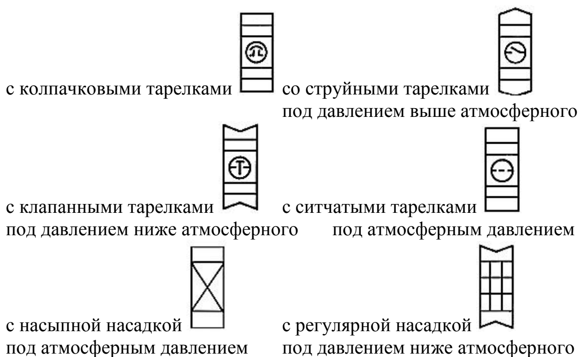
Рис. 2. Обозначения колонных аппаратов
