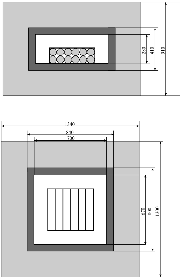
Рис. 1. Эскиз печи
