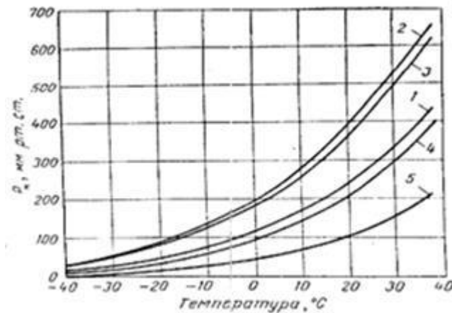
Рис. 1. Влияние температуры на давление насыщенных паров: 1 – А-76; 2,3 – А-76 северный; 4 – Аи-92 летний; 5 – А-76 южный
