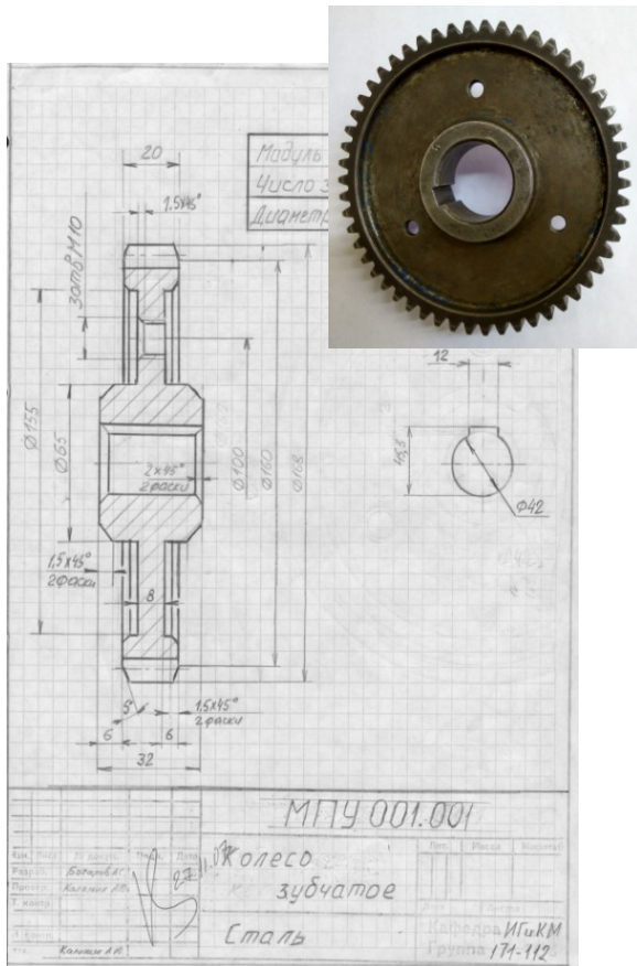
– Эскиз шестерни
