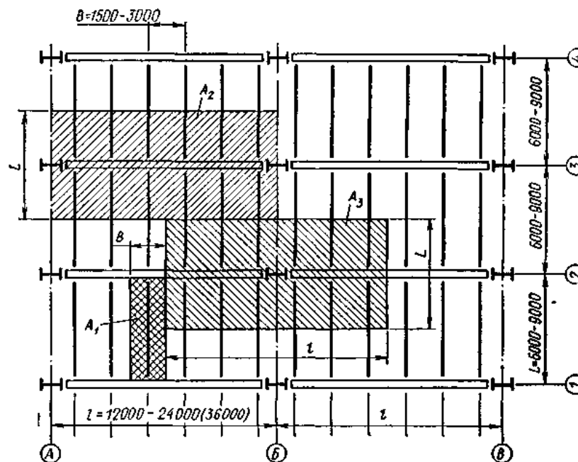
Рис. 1. Балочная клетка:
