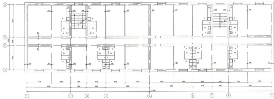
План типового этажа 7
