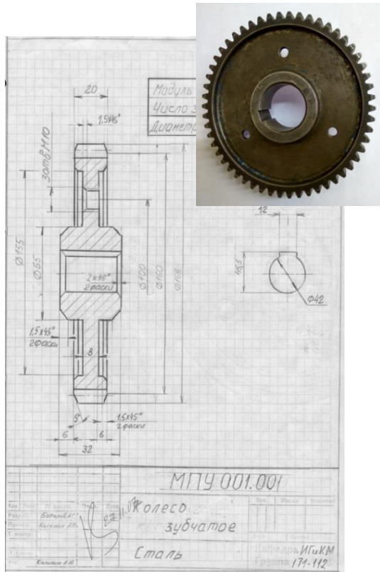
– Эскиз шестерни
