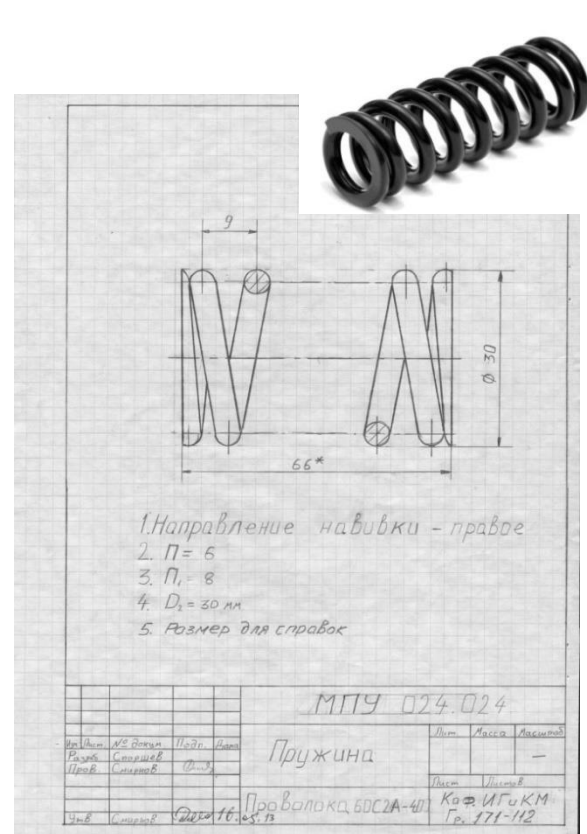
– Эскиз пружины
