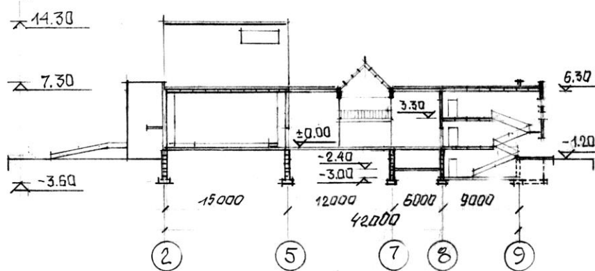
Разрез А-А
