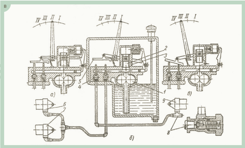
Схема навесной гидросистемы с шестеренчатым насосом
