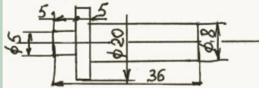
Валик стеклоподъёмника кабины грузовика ЗИС-150
