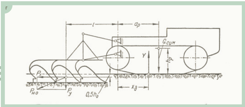
Схема гусеничного трактора с навесными орудиями в рабочем положении (при пахоте)
