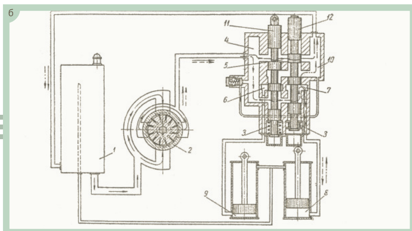
Схема навесной гидросистемы с лопастным насосом
